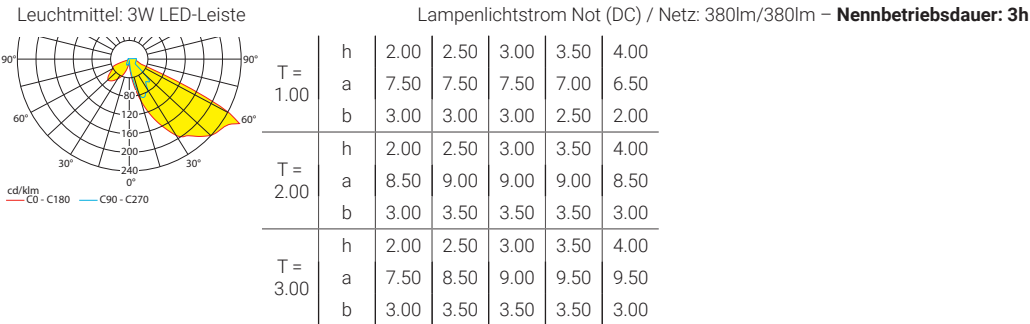
Abstandstabelle ebene Fluchtwege / Tabellenangaben in Meter
